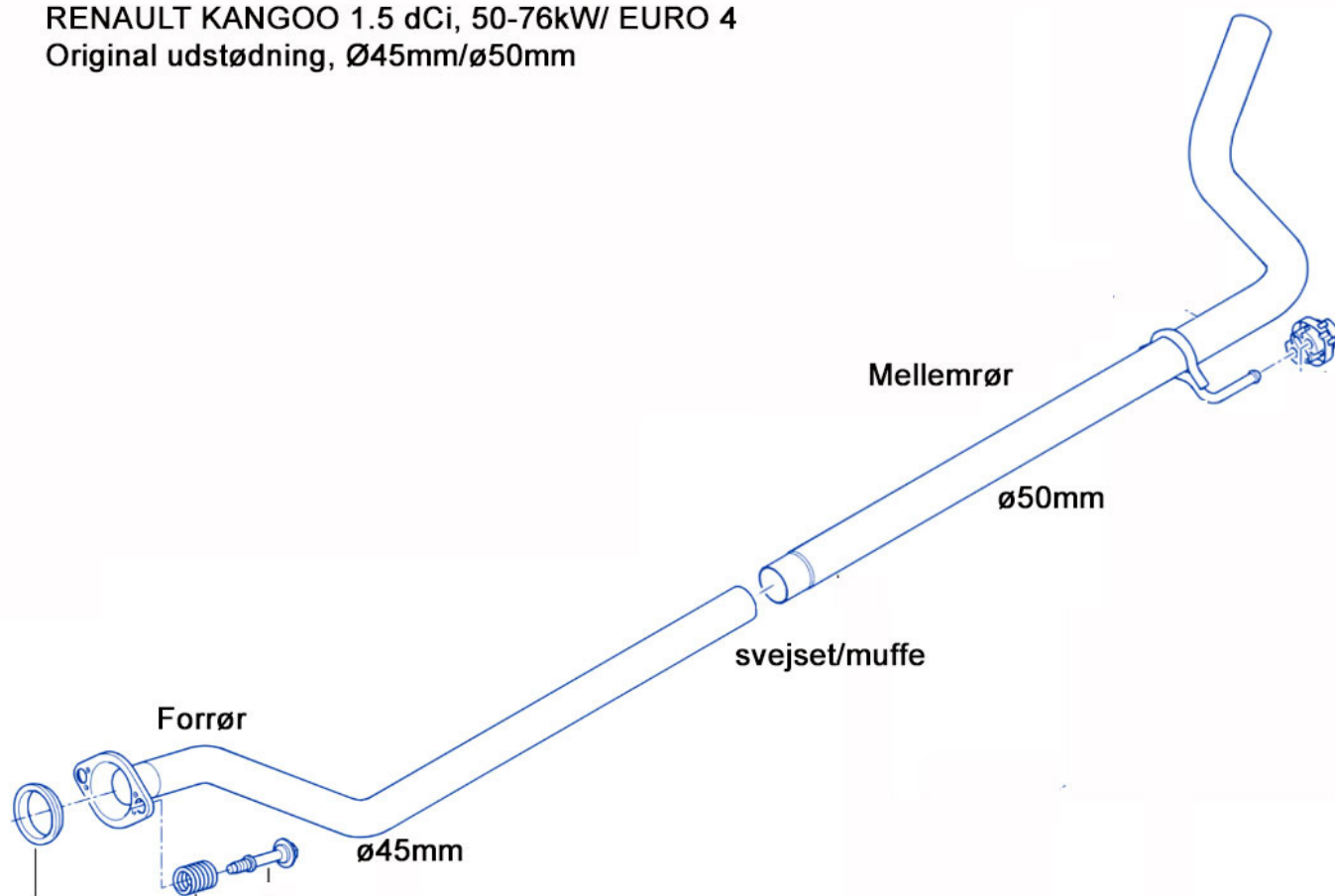
DPF-09 med \varnothing 45\text{mm} studs ind/ \varnothing 50\text{mm} studs ud, 2 clamps og ABE godkendelse.
